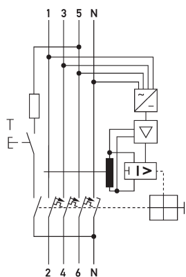
Schaltungsbeispiel FI-/LS-Kombinationen DRCBO 4 Bo6/0,10/3N-B SK
