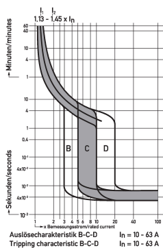
Diagramme Leitungsschutzschalter DLS 6hsl B16-1
