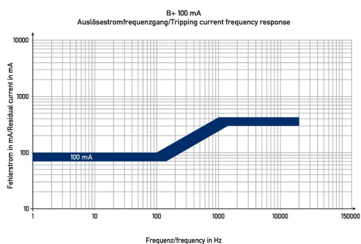
Diagramme FI-/LS-Kombinationen DRCBO 4 B32/0,10/3N-B+
