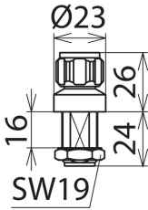
Maßbilder DGA G N
