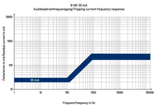
Diagramme FI-/LS-Kombinationen DRCBO 4 C13/0,03/1N-B NK
