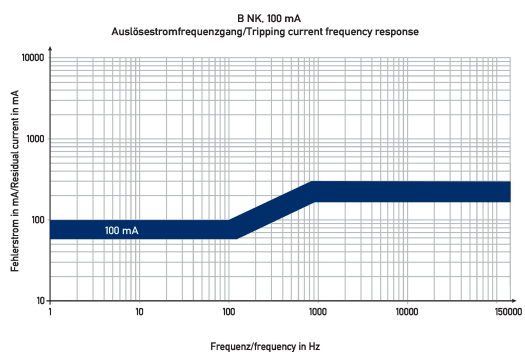
Diagramme FI-/LS-Kombinationen DRCBO 4 Co6/0,10/1N-B NK
