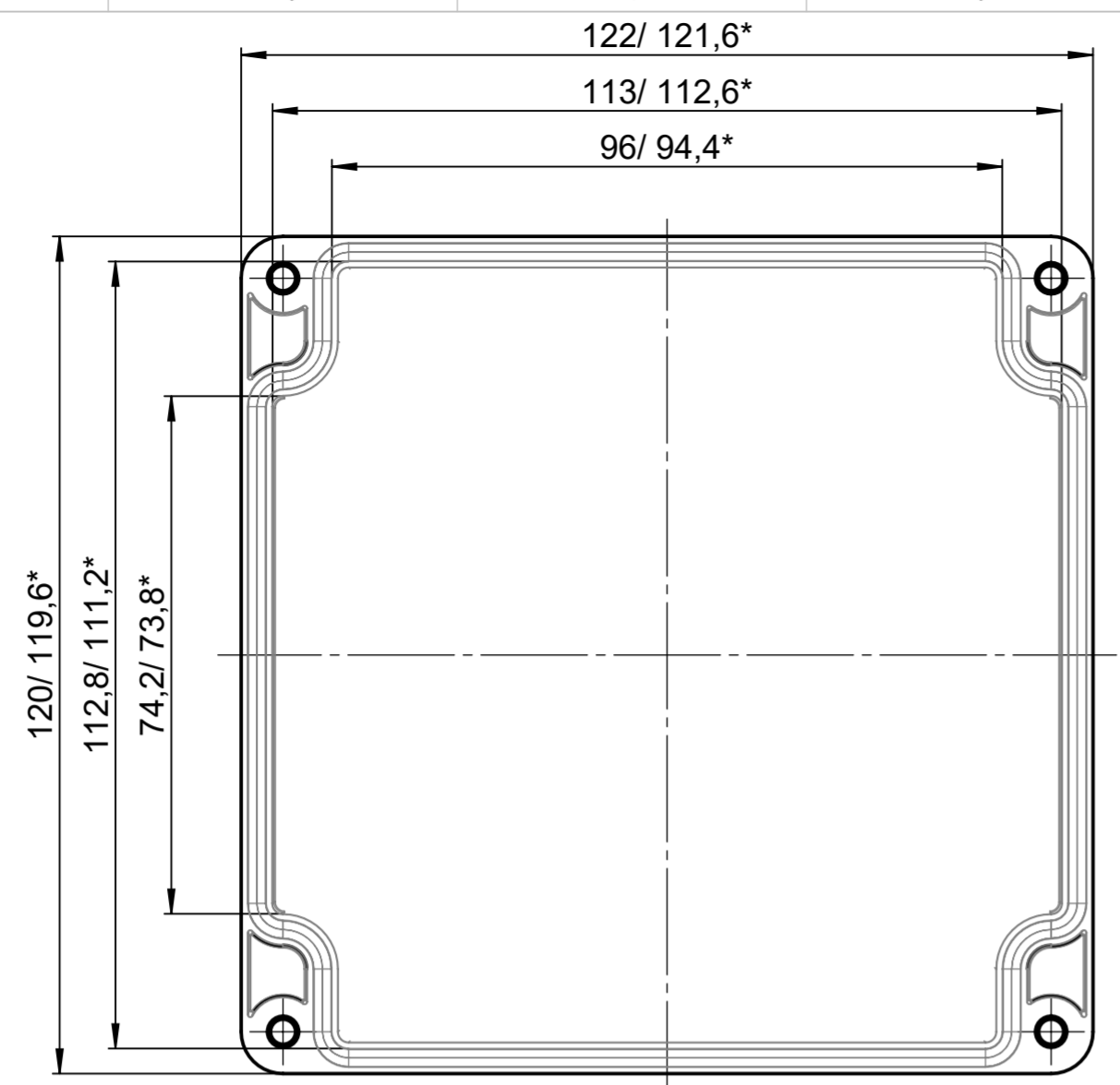
Deckel / Lid
