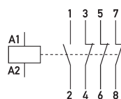
Schaltungsbeispiel Installationsschütze HS 2-024AC/24-13
