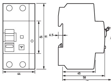
Maßzeichnung FI-/LS-Kombinationen DRCBO 4 C32/0,30/1N-B+
