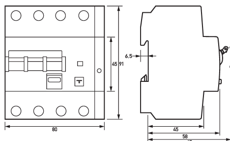
Maßzeichnung FI-/LS-Kombinationen DRCBO 4 C10/0,03/3N-B SK
