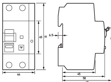
Maßzeichnung FI-/LS-Kombinationen DRCBO 4 Co6/0,03/1N-B+
