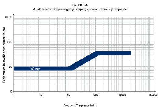
Diagramme FI-/LS-Kombinationen DRCBO 4 C25/0,10/1N-B+
