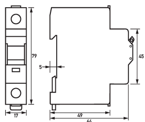
Maßzeichnung Lasttrennschalter RH 063-100
