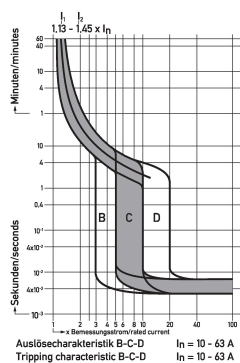
Diagramme Leitungsschutzschalter DLS 6h C16-2
