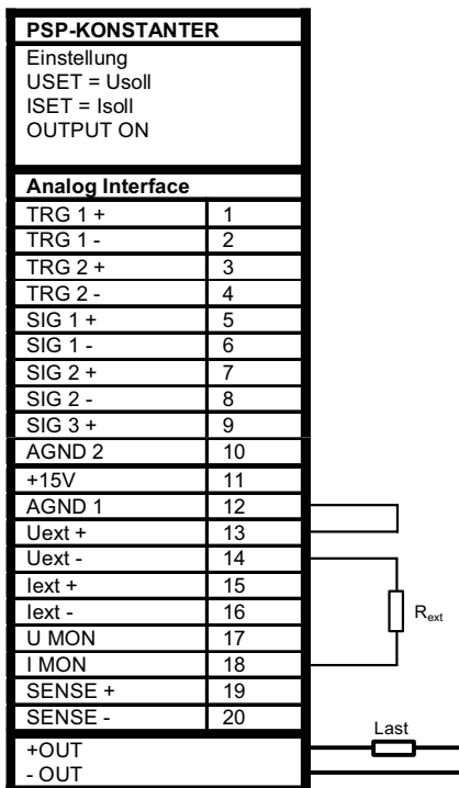
Bild 7.11b Verdrahtung zum Variieren des Innenwiderstandes.
