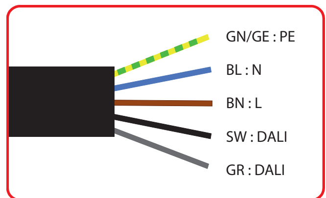
Abb. 7: Anschluss-Diagramm. Die schwarze und graue Ader sind bei Leuchten ohne DALI Funktion zu isolieren. GN/GE: grün/gelb; BL: blau; BN: braun; SW: schwarz
