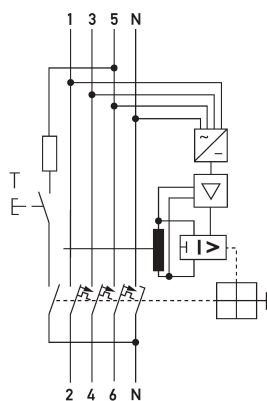
Schaltungsbeispiel FI-/LS-Kombinationen DRCBO 4 Co6/0,30/3N-B NK
