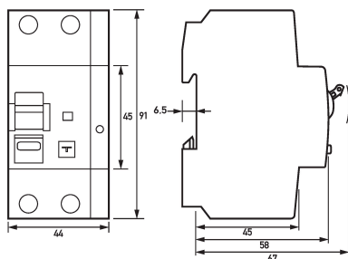
Maßzeichnung FI-/LS-Kombinationen DRCBO 4 Bo6/0,30/1N-B NK
