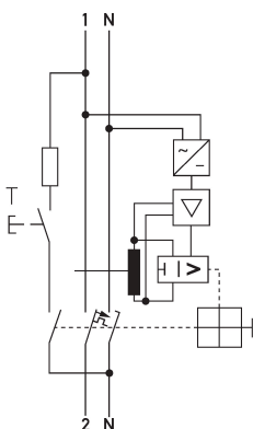
Schaltungsbeispiel FI-/LS-Kombinationen DRCBO 4 Bo6/0,30/1N-B NK
