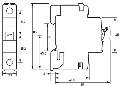
Maßzeichnung Leitungsschutzschalter DLS 6hsl C16-1
