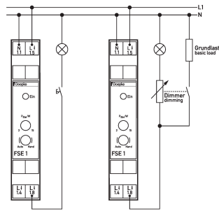
Anschlussschema
