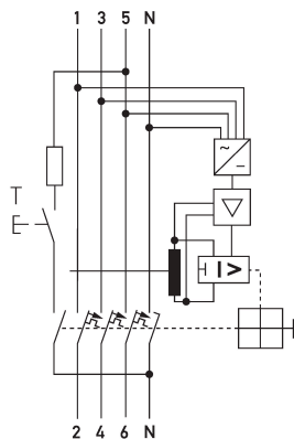
Schaltungsbeispiel FI-/LS-Kombinationen DRCBO 4 C16/0,30/3N-B+
