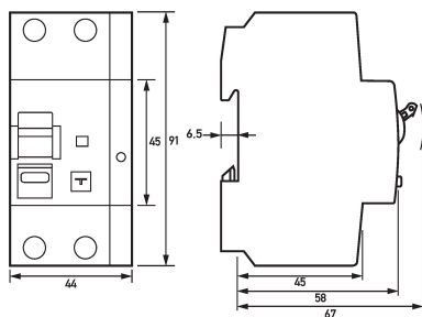
Maßzeichnung FI-/LS-Kombinationen DRCBO 4 C20/0,03/1N-B NK
