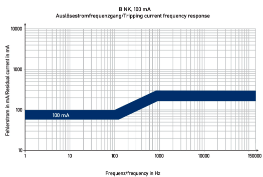
Diagramme FI-/LS-Kombinationen DRCBO 4 C20/0,10/1N-B NK
