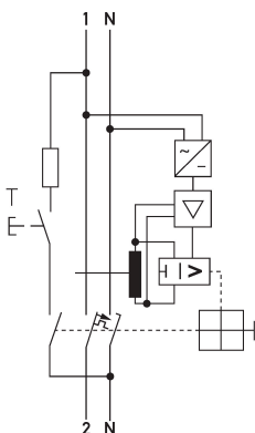
Schaltungsbeispiel FI-/LS-Kombinationen DRCBO 4 C20/0,10/1N-B NK
