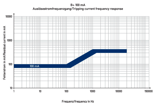
Diagramme FI-/LS-Kombinationen DRCBO 4 C10/0,10/3N-B+
