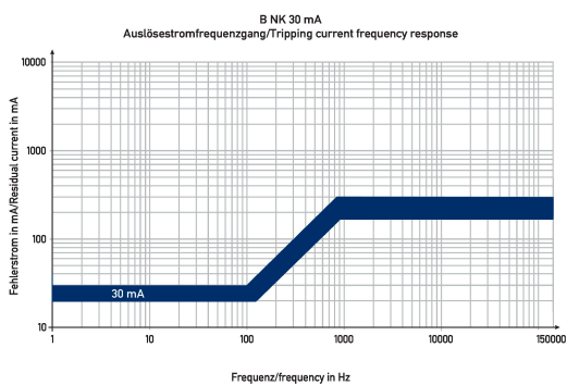
Diagramme FI-/LS-Kombinationen DRCBO 4 B13/0,03/1N-B NK
