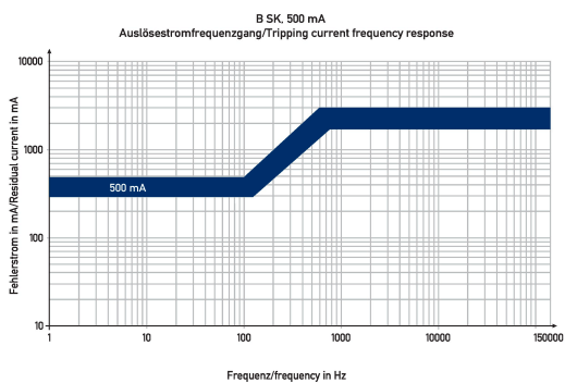
Diagramme Fehlerstromschutzschalter DFS 4 040-4/0,50-B SK R
