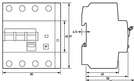
Maßzeichnung FI-/LS-Kombinationen DRCBO 4 Bo6/0,30/3N-B SK
