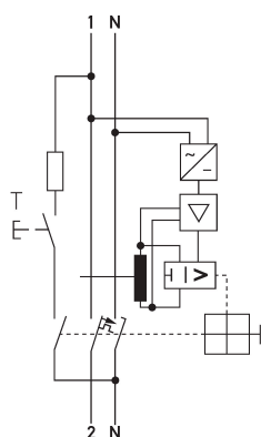
Schaltungsbeispiel FI-/LS-Kombinationen DRCBO 4 B13/0,03/1N-B SK
