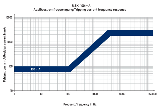
Diagramme FI-/LS-Kombinationen DRCBO 4 B13/0,10/1N-B SK
