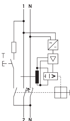
Schaltungsbeispiel FI-/LS-Kombinationen DRCBO 4 B13/0,10/1N-B SK
