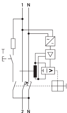
Schaltungsbeispiel FI-/LS-Kombinationen DRCBO 4 B16/0,10/1N-B+
