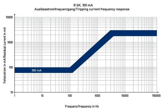
Diagramme FI-/LS-Kombinationen DRCBO 4 Co6/0,10/3N-B SK
