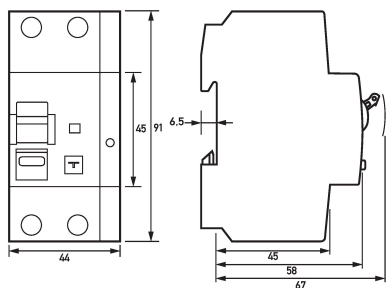
Maßzeichnung FI-/LS-Kombinationen DRCBO 4 Co6/0,10/1N-B NK
