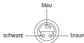
Ansicht auf Steckerstifte
