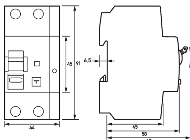
Maßzeichnung FI-/LS-Kombinationen DRCBO 4 Bo6/0,10/1N-B+
