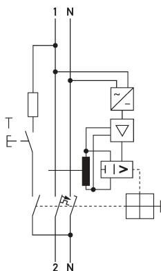
Schaltungsbeispiel FI-/LS-Kombinationen DRCBO 4 Bo6/0,10/1N-B+
