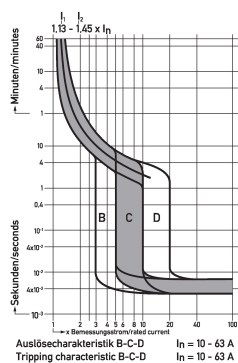
Diagramme Leitungsschutzschalter DLS 6h C20-3+N
