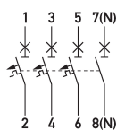
Schaltungsbeispiel Leitungsschutzschalter DLS 6h C20-3+N
