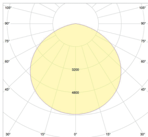
SUN 840 Polardiagramm
