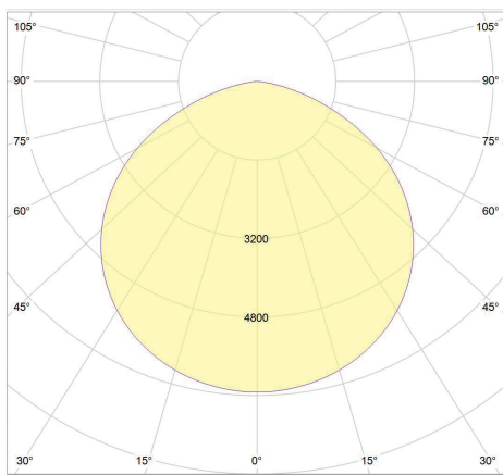
SUN 860 Polardiagramm
