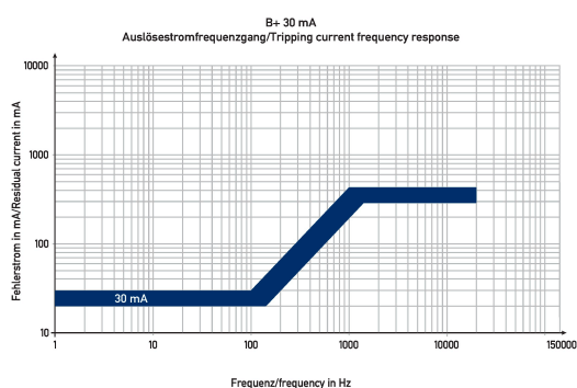
Diagramme FI-/LS-Kombinationen DRCBO 4 B16/0,03/1N-B+
