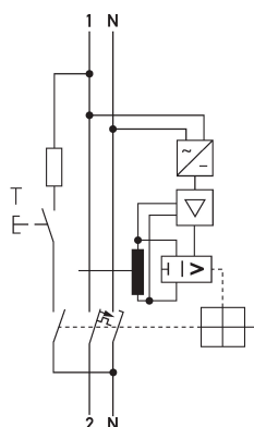
Schaltungsbeispiel FI-/LS-Kombinationen DRCBO 4 B16/0,03/1N-B+
