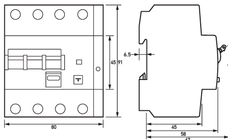
Maßzeichnung FI-/LS-Kombinationen DRCBO 4 Bo6/0,10/3N-B SK
