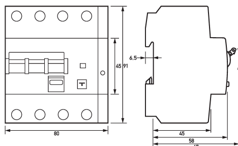
Maßzeichnung FI-/LS-Kombinationen DRCBO 4 Co6/0,10/3N-B+
