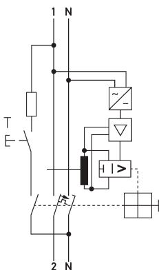
Schaltungsbeispiel FI-/LS-Kombinationen DRCBO 4 C16/0,10/1N-B+
