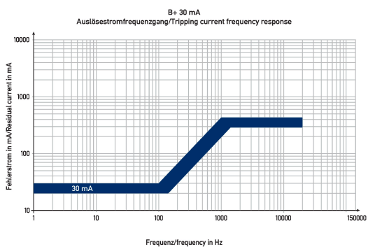
Diagramme FI-/LS-Kombinationen DRCBO 4 C20/0,03/1N-B+
